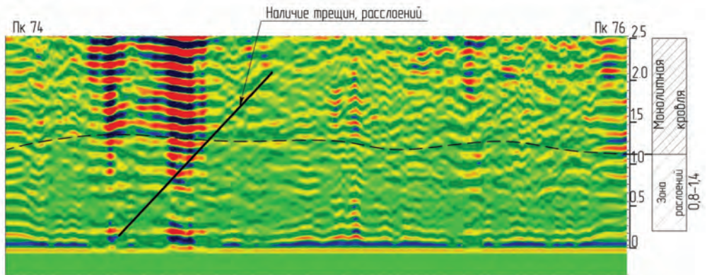
Рис. 2. Георадарограмма кровли, трасса № 2, антенна 400 МГц, зона отслоившейся кровли 0,8–1,4 м, относительно равномерная по толщине, наблюдаются признаки наличия трещин в кровле, виден влагонасыщенный участок
