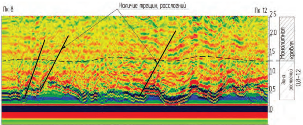
Рис. 1. Георадарограмма кровли, трасса № 1, антенна 400 МГц, зона отслоившейся кровли 0,8–1,2 м, относительно равномерная по толщине, наблюдаются признаки наличия трещин в кровле
