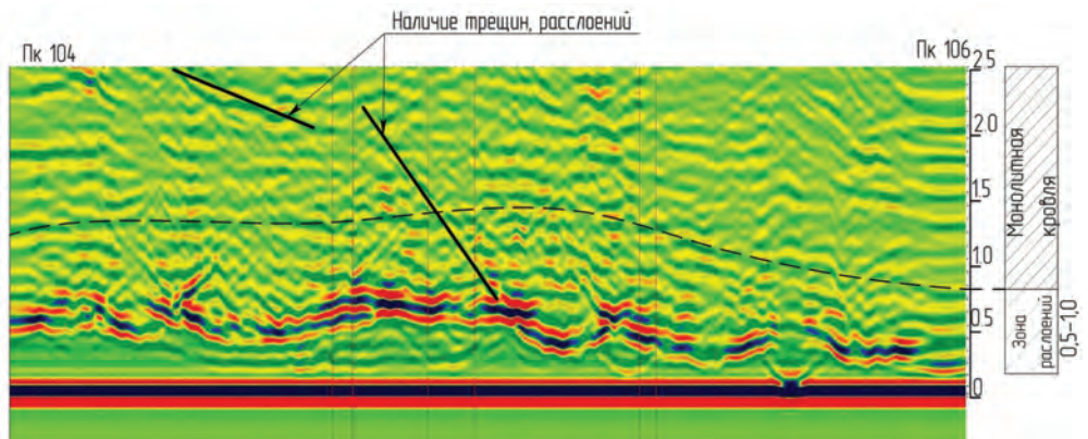
Рис. 3. Георадарограмма кровли, трасса № 3, антенна 400 МГц, зона отслоившейся кровли 0,5–1,0 м, неравномерная по толщине, наблюдаются признаки наличия череды трещин в кровле, способствующие появлению вывалов
