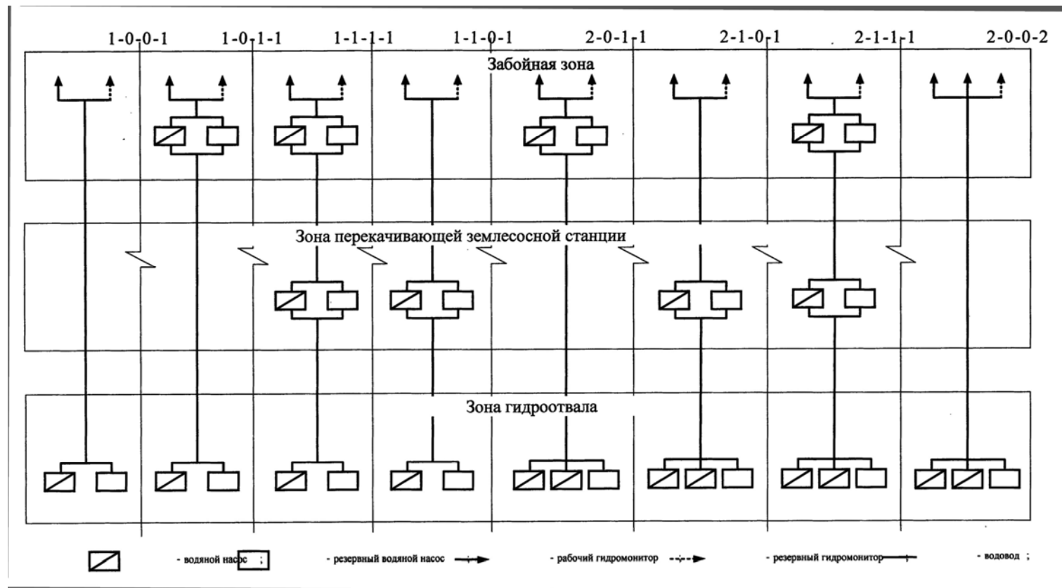
Рис. 3. Типовые структуры насосно-гидромониторных установок
