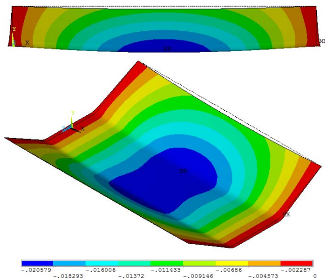
Рис. 5. Деформации конвейерной ленты между роликкооперами
