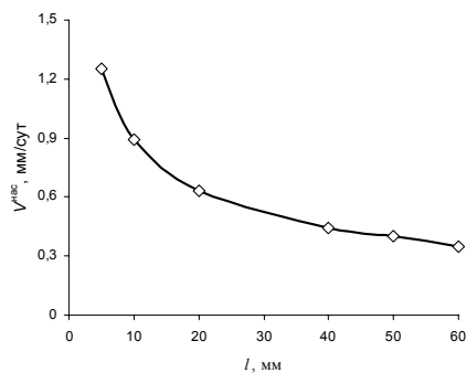
Рис. 3. Зависимость скорости насыщения ( V^{нас} ) от глубины насыщения ( l ) для n = 25.1-27.0\% .
