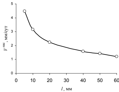
Рис. 6. Зависимость скорости насыщения ( V^{нас} ) от глубины насыщения ( l ) для n > 35\% .
