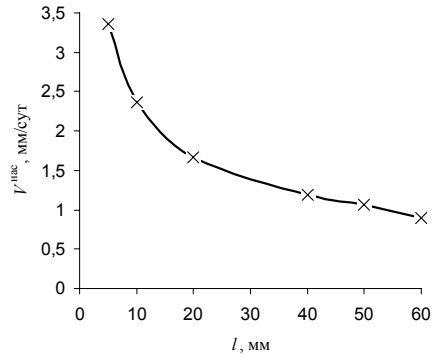
Рис. 5. Зависимость скорости насыщения ( V^{нас} ) от глубины насыщения ( l ) для n = 31.1-35\% .
