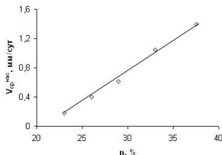
Рис. 8. Зависимость средних скорости насыщения куска ( V_{ср}^{нас} ) от общей пористости ( n ) и глубины проработки 20-70 мм
