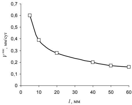
Рис. 2. Зависимость скорости насыщения ( V^{нас} ) от глубины насыщения ( l ) для n \leq 25\% .
