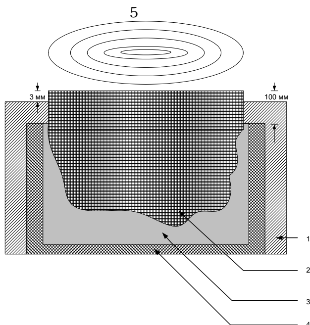
Рис. 1. Лабораторная установка для исследования глубины проникания растворов: 1 - выщелачивающий раствор; 2 - рудный кусок; 3 - эпоксидная смола; 4 - деревянная подставка; 5 - концентрические бороздки для замера рН
