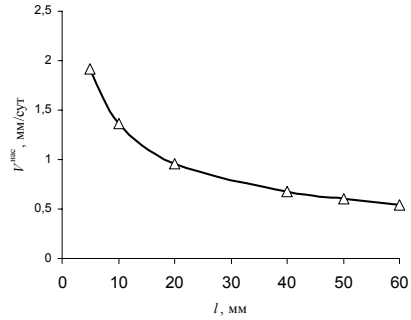
Рис. 4. Зависимость скорости насыщения ( V^{нас} ) от глубины насыщения ( l ) для интервала пористости n = 27.1-31\% .
