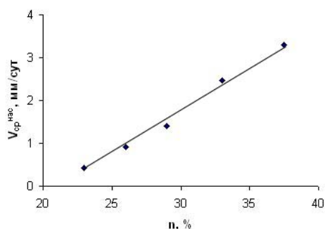
Рис. 7. Зависимость средних скорости насыщения куска ( V_{ср}^{нас} ) от общей пористости ( n ) и глубины проработки < 20 мм
