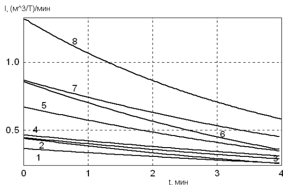
Рис. 6. Скорость изменения содержания метана в образцах угля при десорбции
