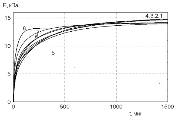
Рис. 5. Характер изменения давления в накопительном сосуде при десорбции метана из угля – образцы №№ 1-8
