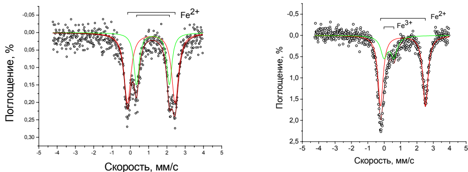
Рис. 2. Мессбауэровские спектры образцов угля: (а) – из спокойной области, (б) – из выбросоопасной зоны.
