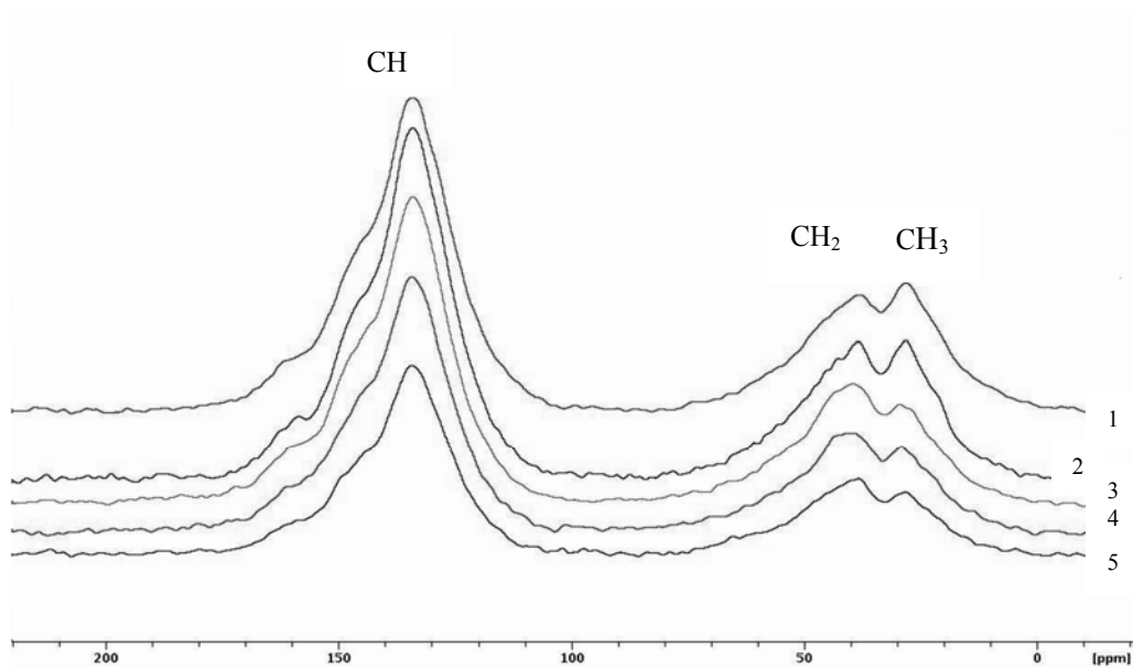
Рис. 3. Спектры ЯМР ^{13}\text{C} CP/MAS образцов углей из пласта h'б ш. им. Скочинского: выбросоопасная зона (1,2), выброс (3), спокойная область (4,5)
