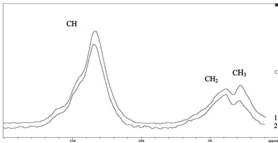
Рис. 4. Спектры ЯМР ^{13}\text{C} CP/MAS образцов углей из пласта h'б ш. им. Скочинского: 1 – выбросоопасная зона 2 – спокойная область
