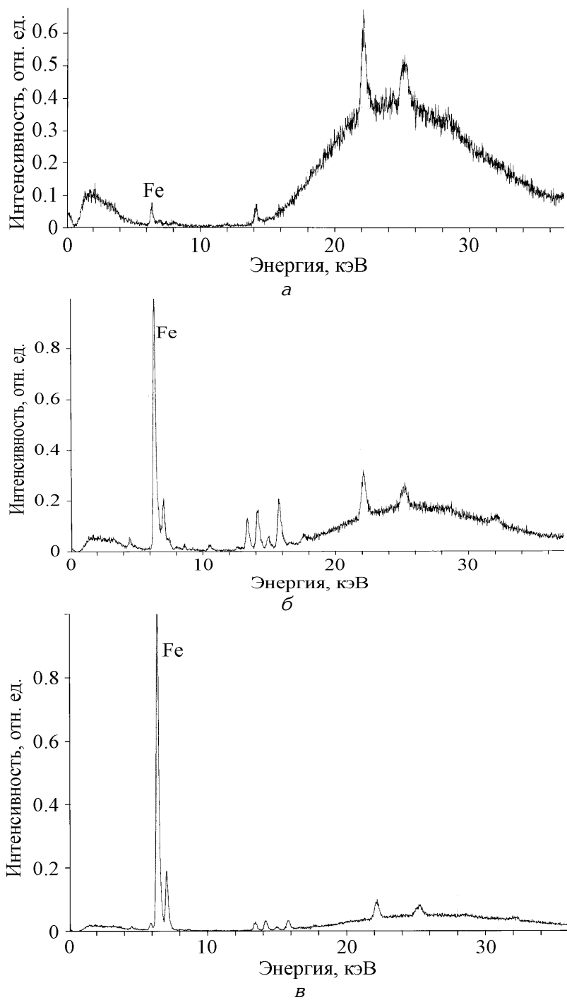
Рис. 1. Рентгенофлуоресцентные спектры образцов: а – № 6 из спокойной области; б – № 34,36 из зоны ГДЯ, происшедшего 19.03.2009 г; в – №25 из выбросоопасной зоны возле ГДЯ, происшедшего 14.03.2009 г.
