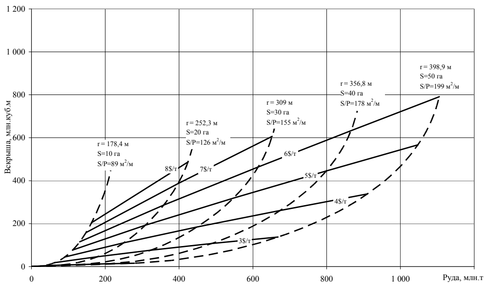
Рис. 9. Зависимости объемов вскрышных пород от запасов руды в контурах карьеров, разрабатывающих штокверковые месторождения с различной горизонтальной мощностью рудного тела
