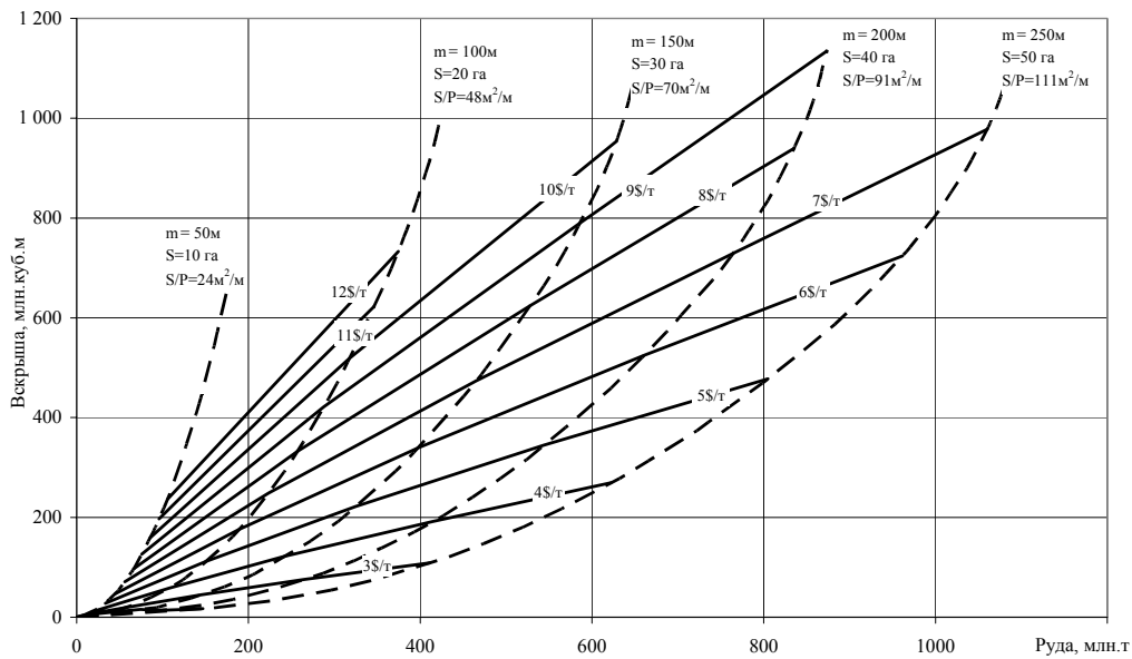
Рис. 8. Зависимости объемов вскрышных пород от запасов руды в контурах карьеров, разрабатывающих пластовые месторождения с различной горизонтальной мощностью рудного тела
