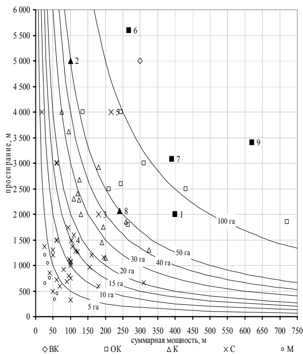
а) распределение месторождений по запасам
