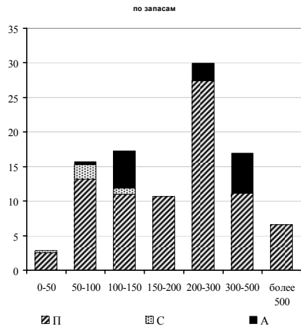
а) б) Рис. 5. Распределение запасов железорудных месторождений разной крупности (а) и разного морфологического строения (б) в зависимости от горизонтальной мощности рудных тел
