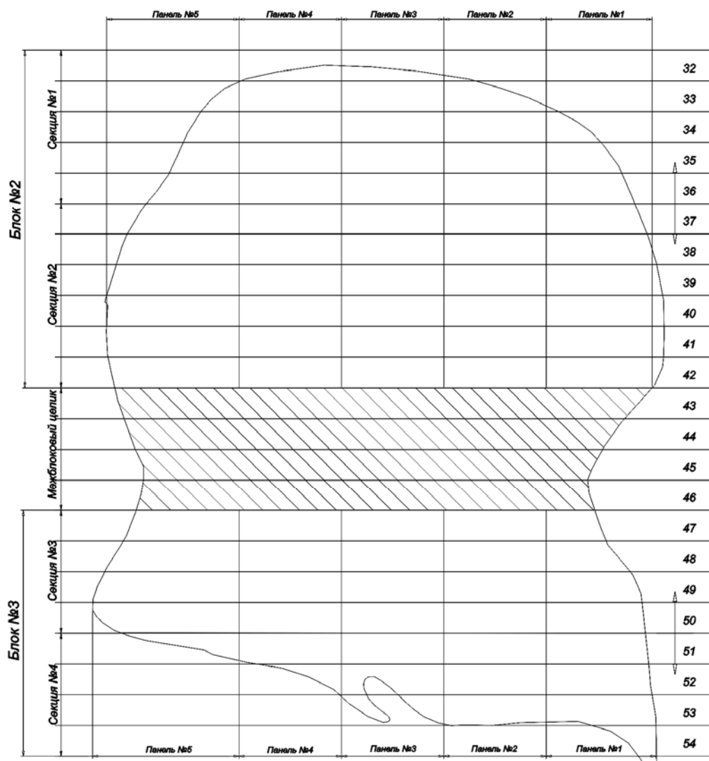
Принципиальная схема разбивки запасов при сплошном порядке отработки
