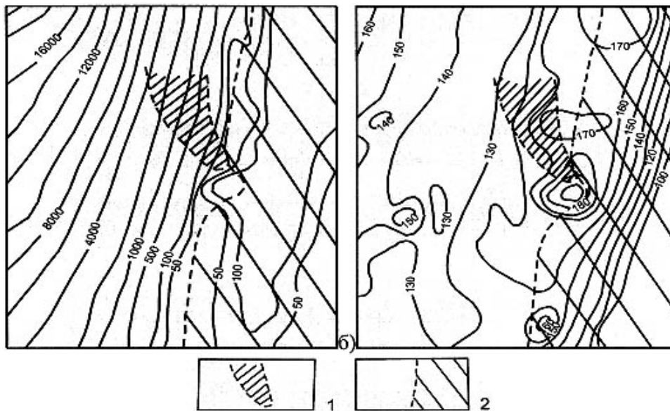
Рис. 2. Распределение удельной энергии деформации (а) — объема, (б) — формы в пределах Естюнинского месторождения: 1 — контур месторождения, 2 — область отрицательных значений дилатации
