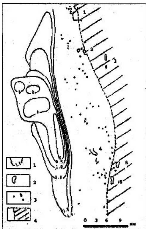
Рис. 1. Морфология Плутона гипербазитов и металлогенические результаты анализа поля деформаций: 1 — изогипсы поверхности Плутона гипербазитов (оцифровка в км); 2 — месторождения; 3 — рудопроявления; 4 — область аномальных значений поля деформаций. Месторождения: 1 — Гороблагодатское; 2 — Валуевское; 3 — Осокино-Александровское; 4 — Естюнинское; 5 — Лебяжинское; 6 — Высокосгорское
