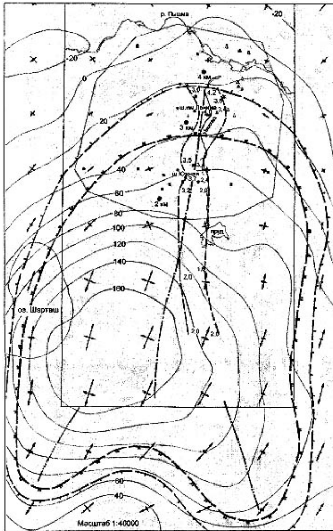
Рис. 4. Деформационная характеристика Березовского золоторудного месторождения: 1 — шахты, рудники; 2 — глубина кровли гранитов по геофизическим данным (в км); 3 — направления растяжения (со стрелками) и сжатия (без стрелок); 4 — контур зоны площадного растяжения (2 штриха) одностороннего растяжения (1 штрих); 5 — оси зоны площадного растяжения первого порядка (одн точка) и второго порядка (2 точки); 6 — изолинии дилатации (в условных единицах); 7 — контур SOH1 пересечения даек с указанием глубин пересечений (в км); 8 — контур зоны промышленного золотого оруденения Березовского рудного поля
