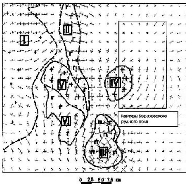
Рис. 3. Поле главных значений тензора чистой деформации района г. Екатеринбурга. Массивы: I — Верх-Исетский; II — Шувакишский; III — Уктусский; IV — Шарташский; V — Свердловский; VI — Ширококоренский
