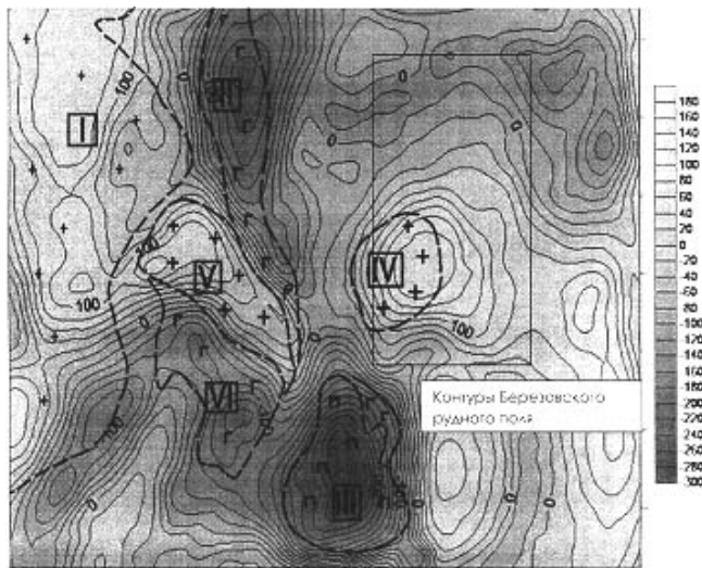
Рис. 5. Поле дилатации района г. Екатеринбурга. Массивы: I — Верх-Исетский; II — Шувакишский; III — Уктисский; IV — Шарташский; V — Свердловский; VI — Ширококореченский
