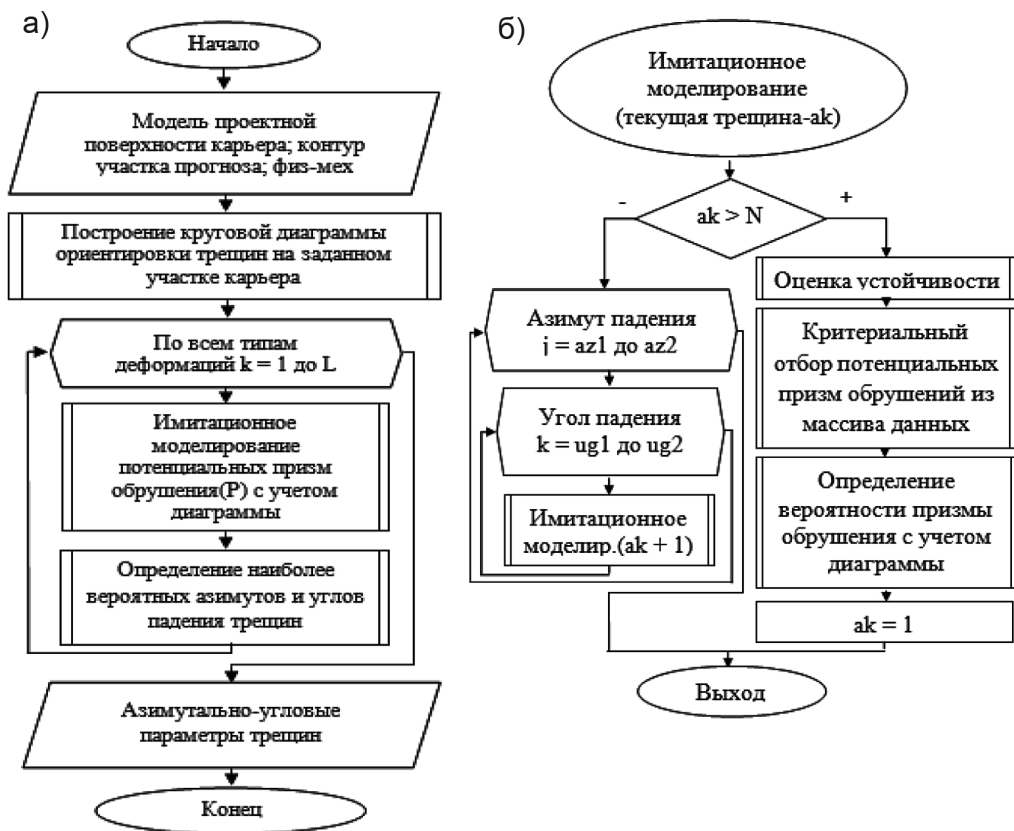
Блок-схемы: алгоритма вероятностного прогноза азимутально-угловых параметров трещин, ограничивающих потенциальные деформации уступов карьера (а); рекурсивного алгоритма имитационного моделирования потенциальных призм обрушения (б)
