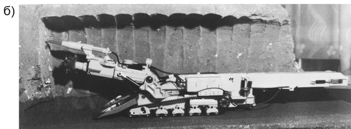
Рис. 2. Модель проходческого комбайна с комбинированным исполнительным органом: режущей головкой и ударным исполнительным органом: а) режущей головкой производится вруб по плитку у почвы выработки, б) ударным рабочим органом разрушается забой над врубом
