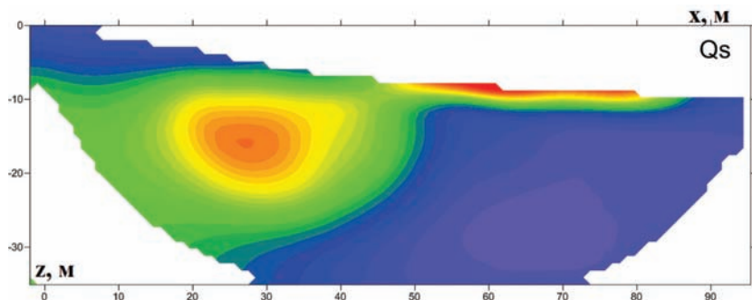
Рис. 3. Сейсмотомографический разрез декремента затухания поперечных волн. В левом углу выделяется ослабленная зона круглого сечения
